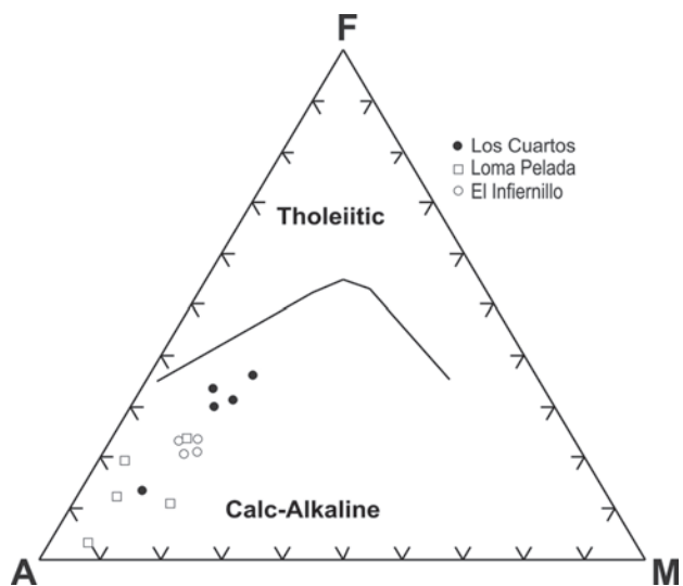
Fig. 3.—Diagrama AFM (Irvine & Baragar, 1971).
