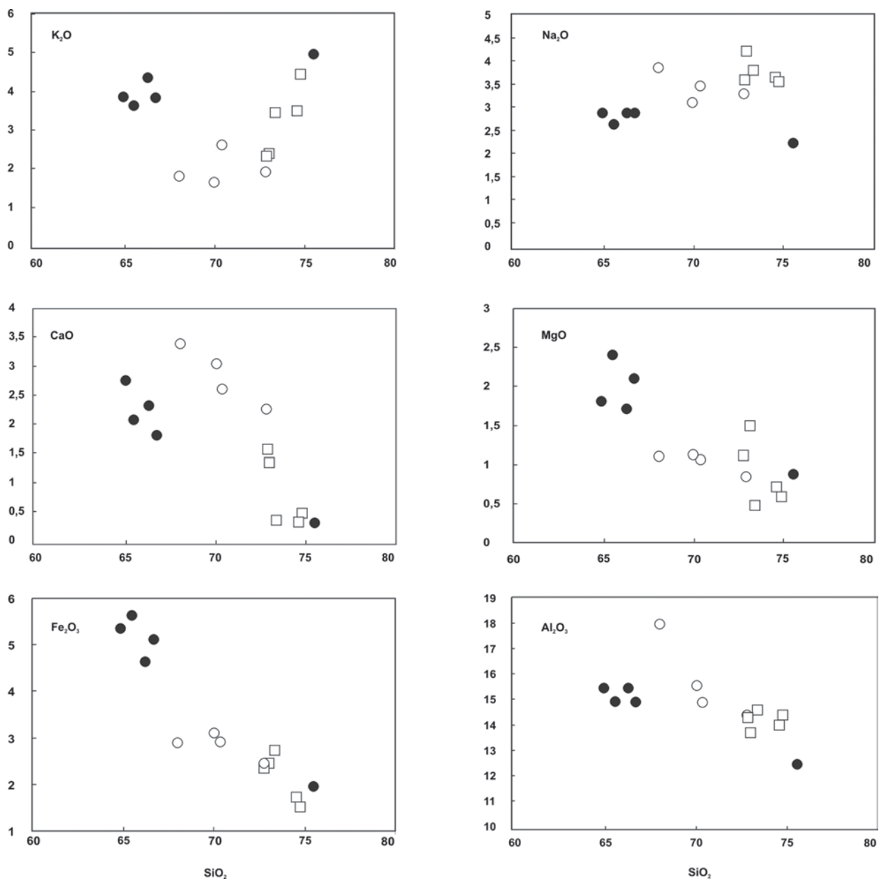
Fig. 6.—Diagramas de variación de elementos mayores vs. SiO 2 .
