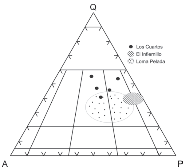
Fig. 2.—Diagrama QAP de Streckeisen (1976) con la proyección de las rocas estudiadas.
