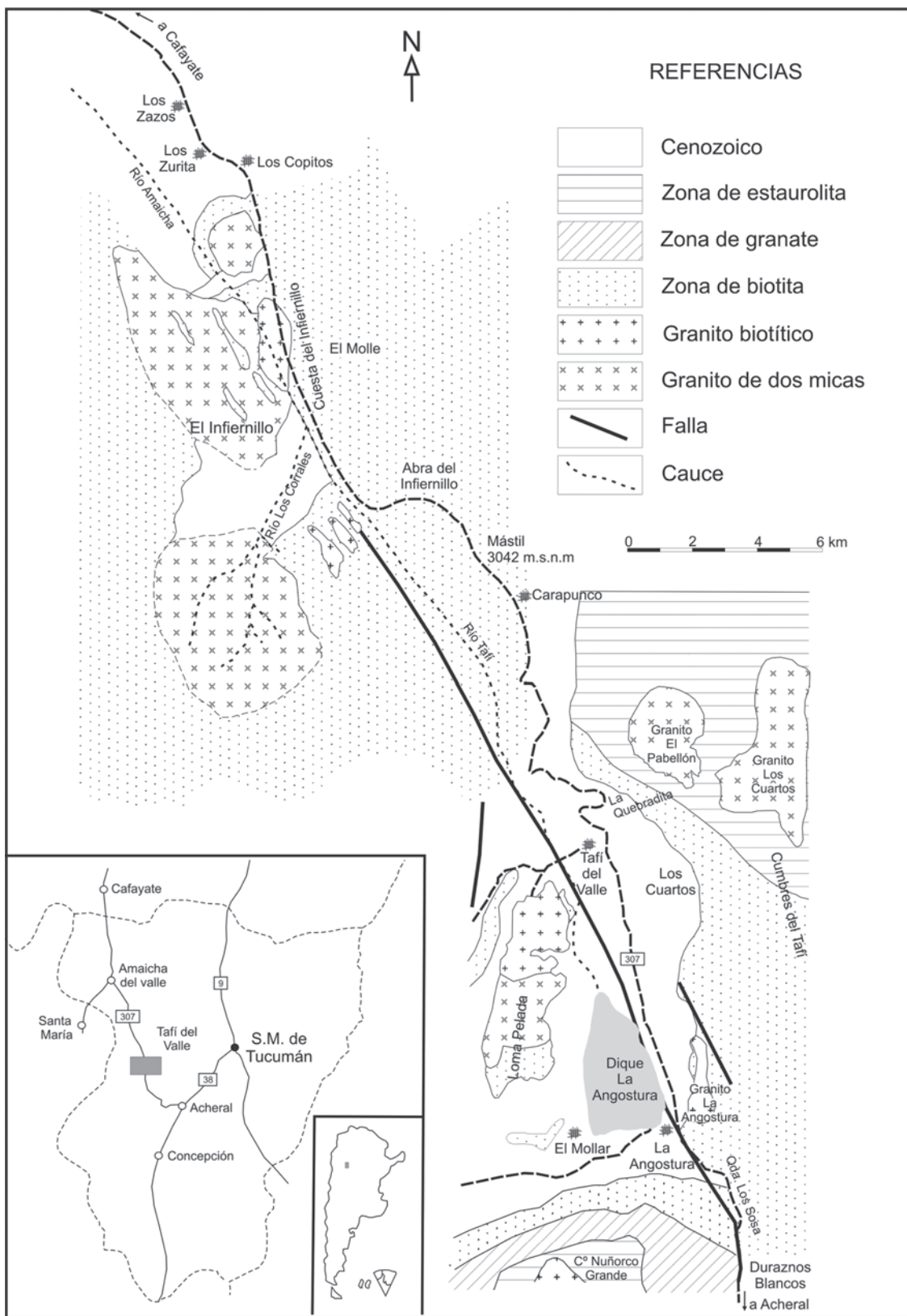
Fig. 1.—Esquema geológico de la zona de estudio.
