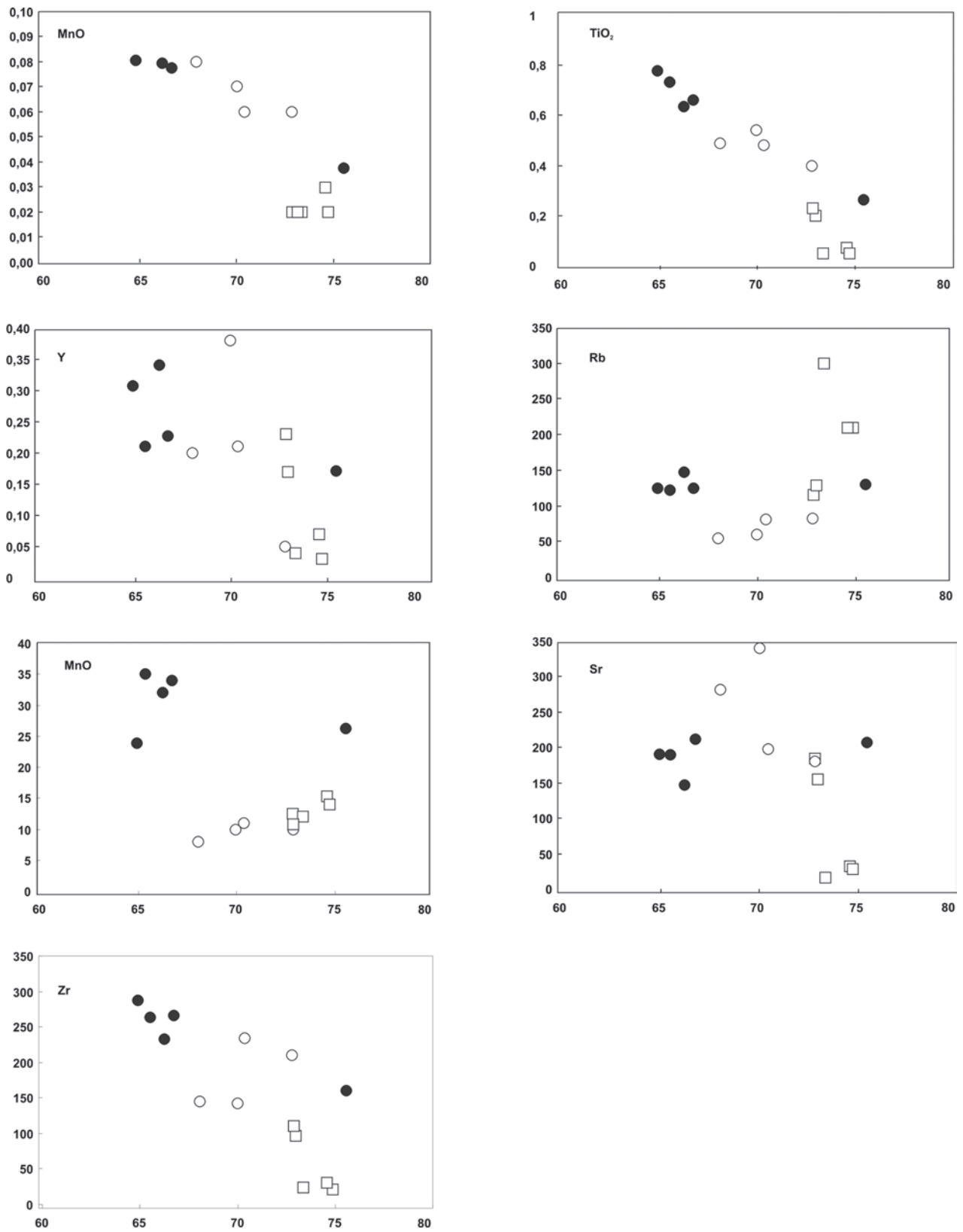
Fig. 7.—Diagramas de variación de elementos menores y trazas vs. SiO 2 .
