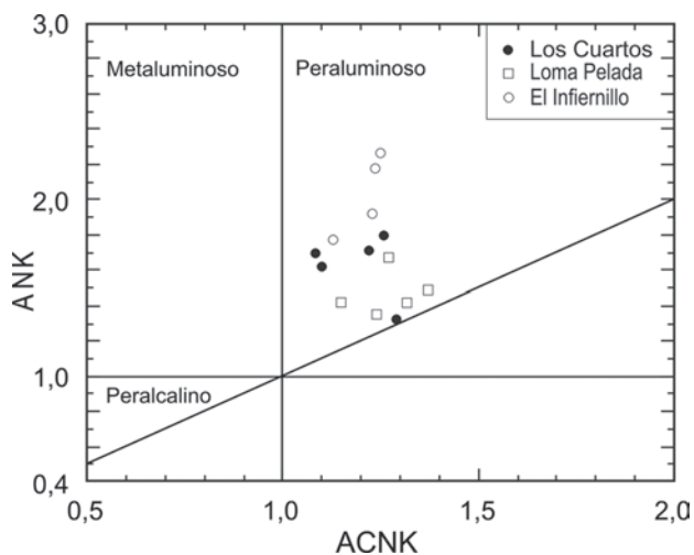
Fig. 4.—Diagrama de Maniar & Piccoli (1989) utilizando los índices de Shand.
