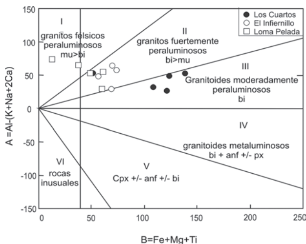
Fig. 5.—Diagrama de discriminación de Debon & Le Fort (1983).
